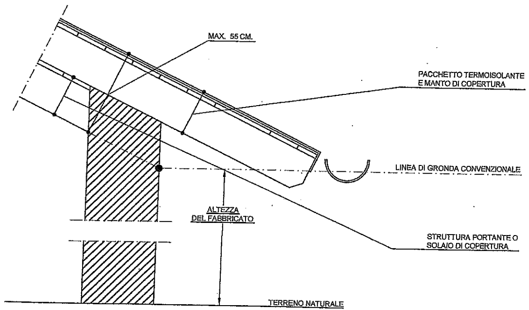
NORMA IN VIGORE (ART. 3 COMMA 6 DEL N.T.A.) - COPERTURA TIPO "FASSA"
