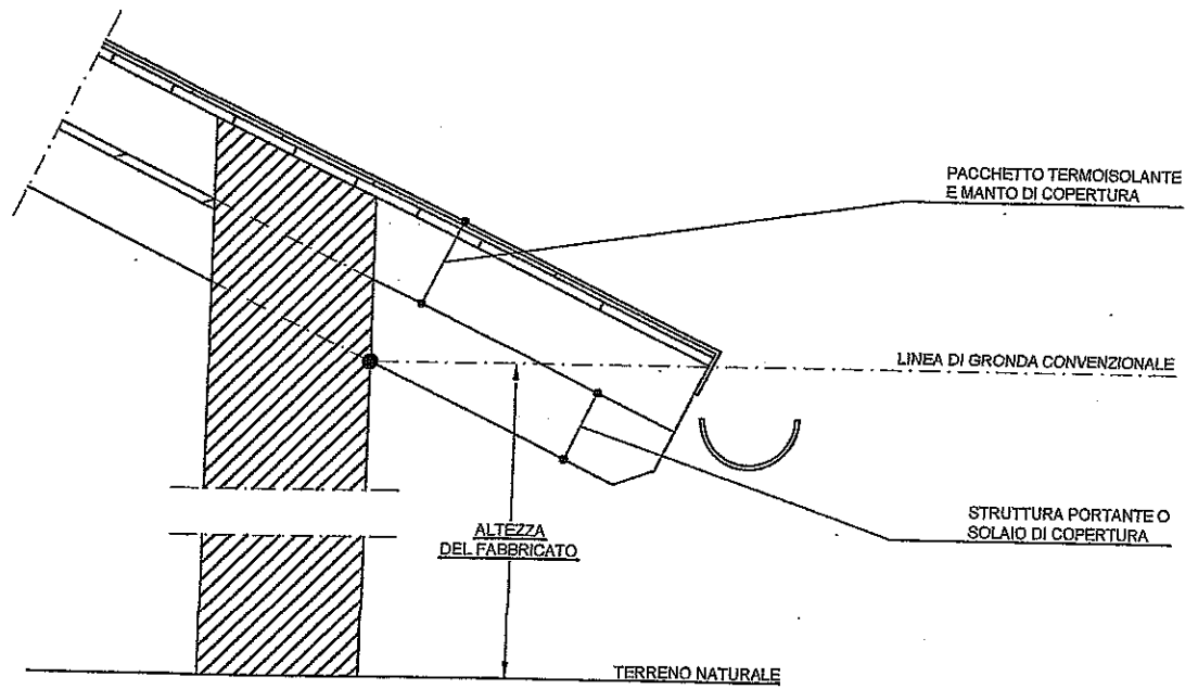
NORMA IN VIGORE (ART. 3 COMMA 6 DEL N.T.A.) - COPERTURA TRADIZIONALE
